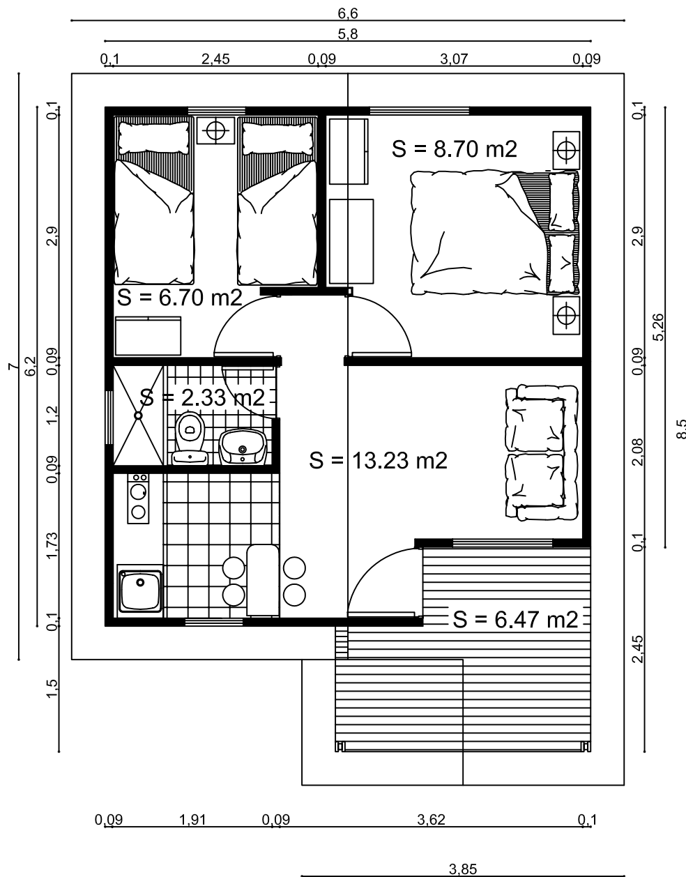
PLANTA
