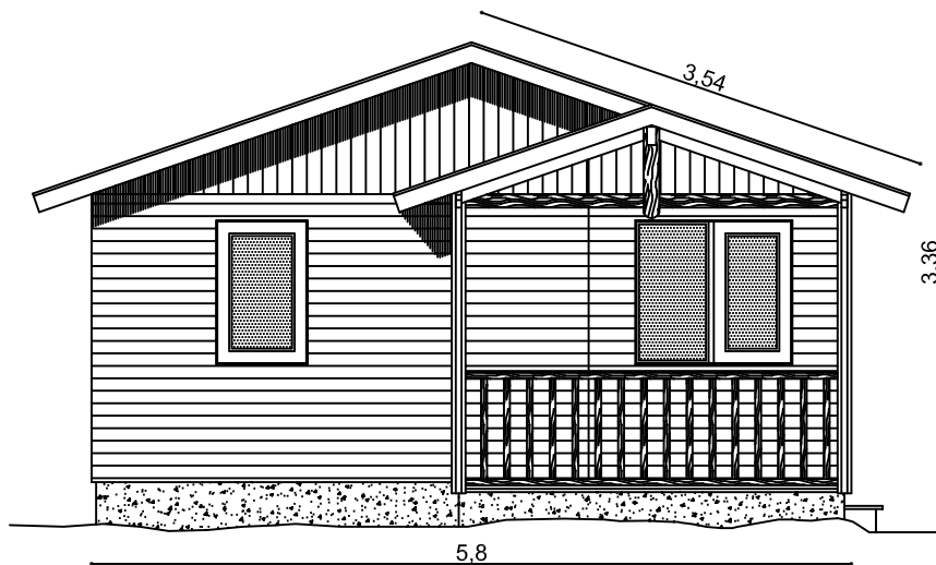
ALZADO
