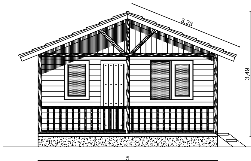
ALZADO
