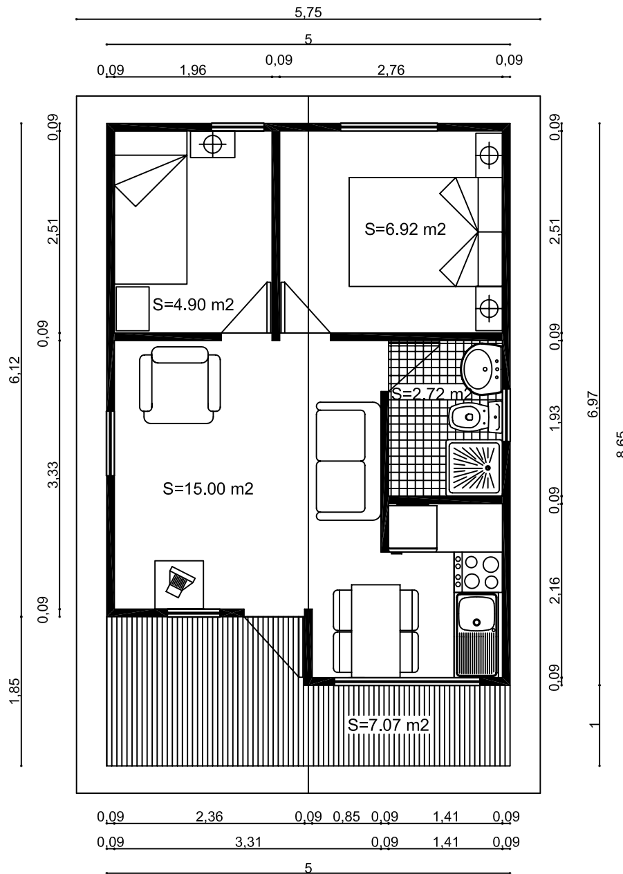
PLANTA
