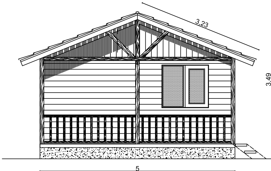
ALZADO
